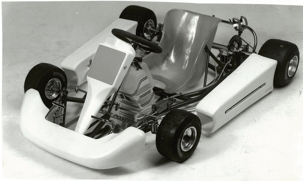
Photo du châssis avec pneumatique
